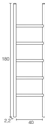
ESCALERA VELVET A ÉCHELLE VELVET A LADDER VELVET A
