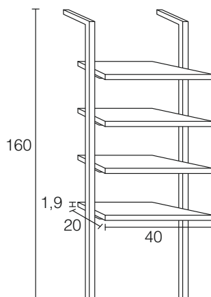
ESCALERA VELVET B ÉTAGÈRE VELVET B LADDER VELVET B
